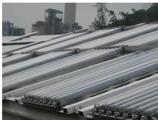
太阳能热水系统
